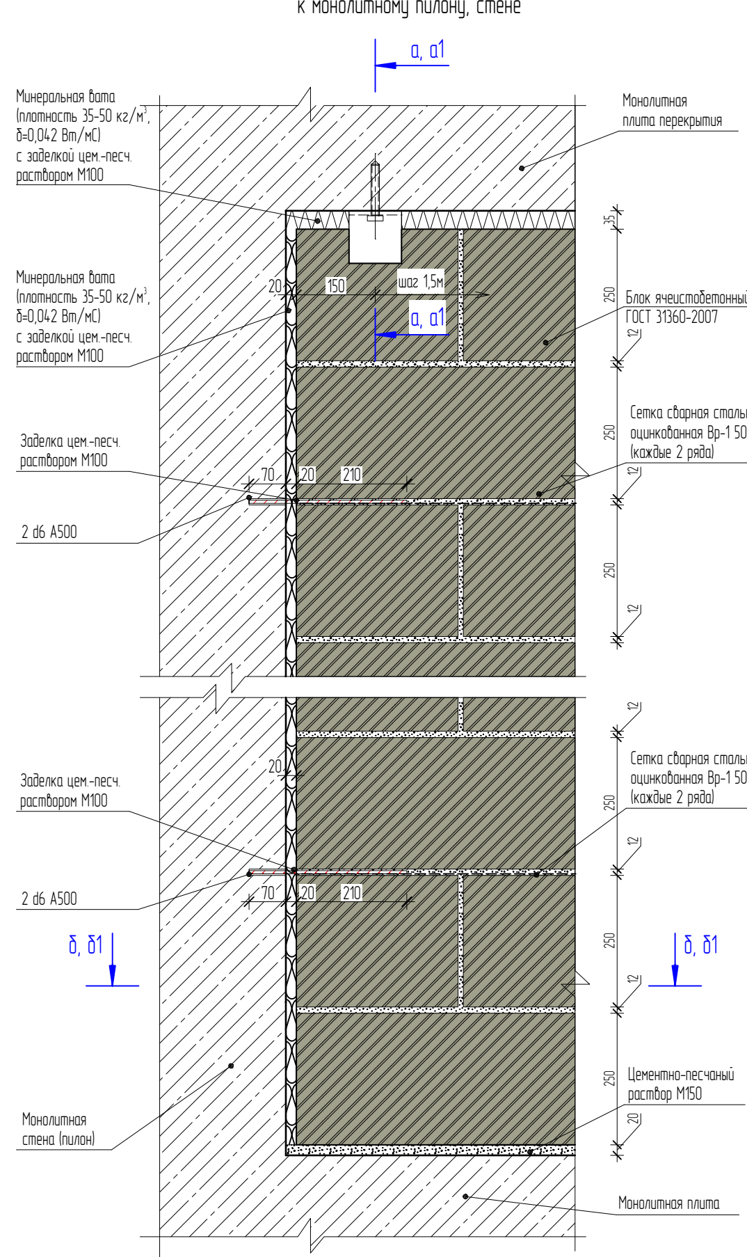
Вид А М110
