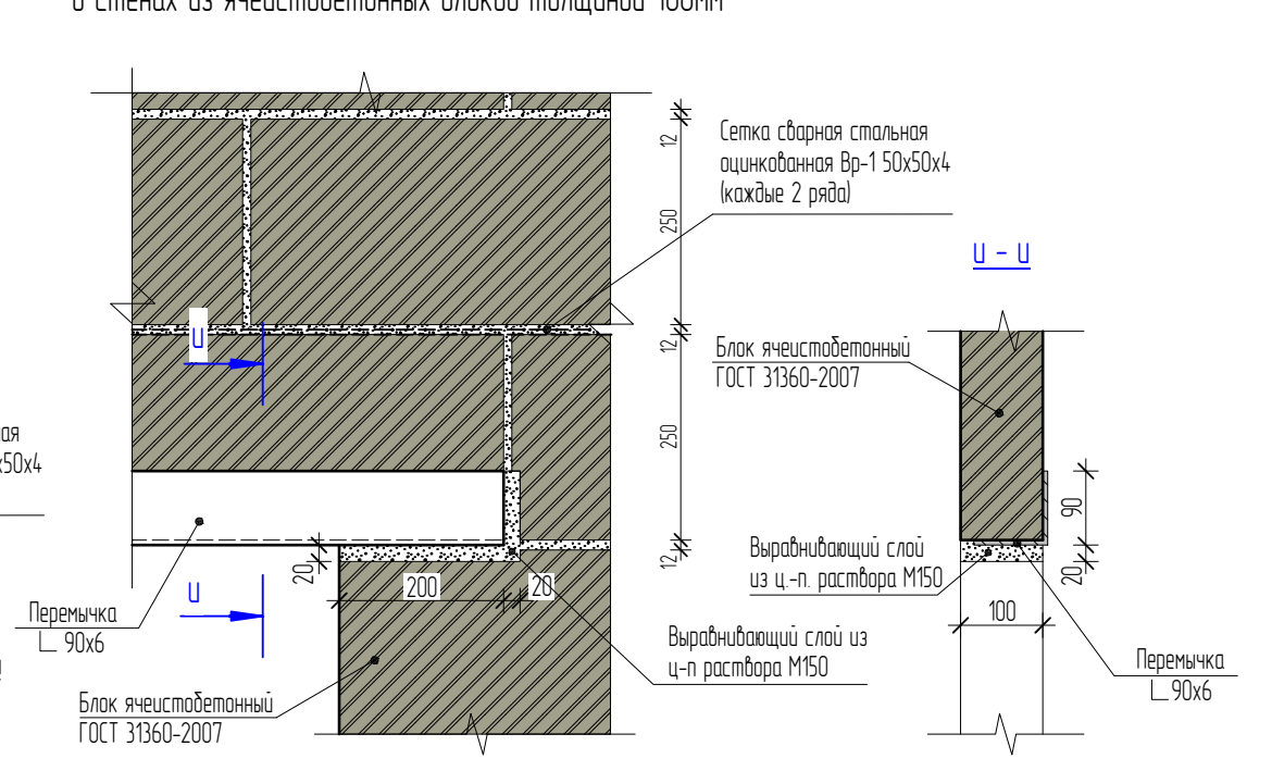
Вид Д1 М110
