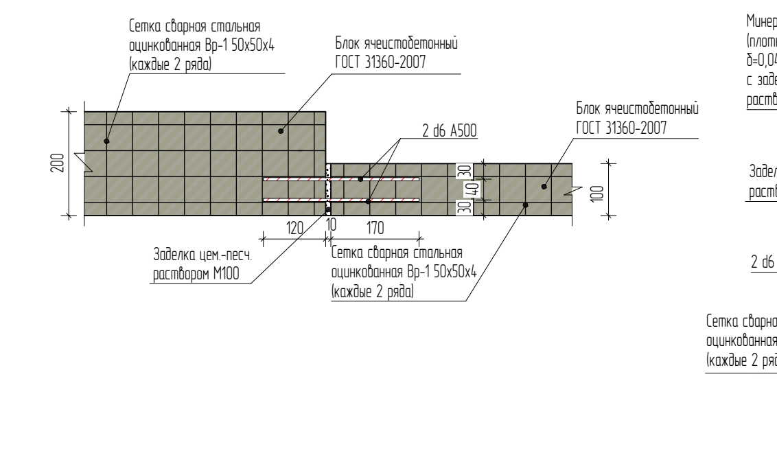
Вид Г М110
