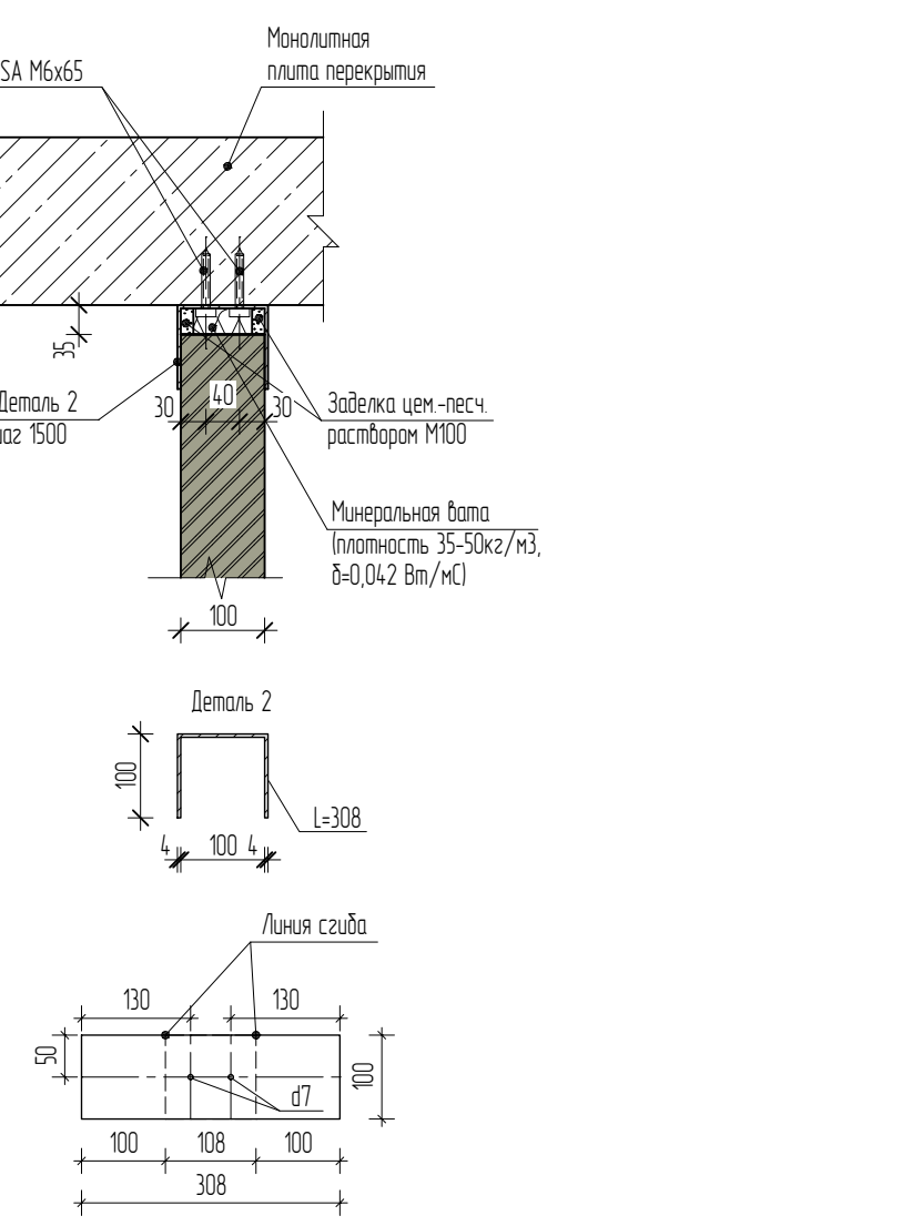
а1 - а1
