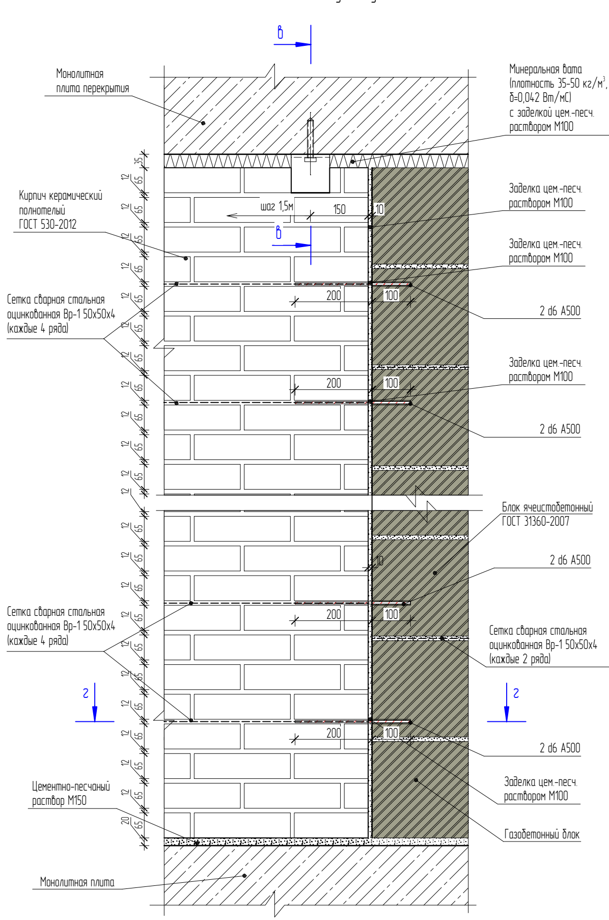
Вид Д3 М110
