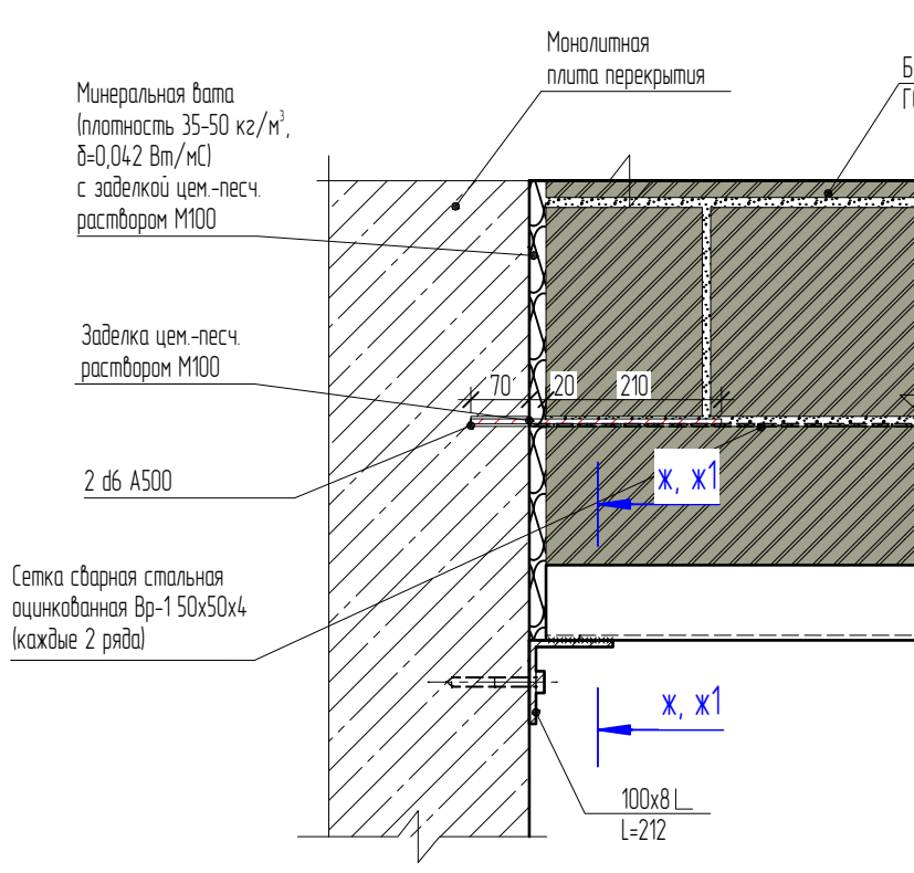
Вид Д3 М110
