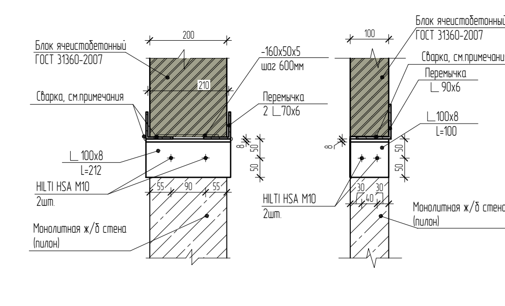
х - х
