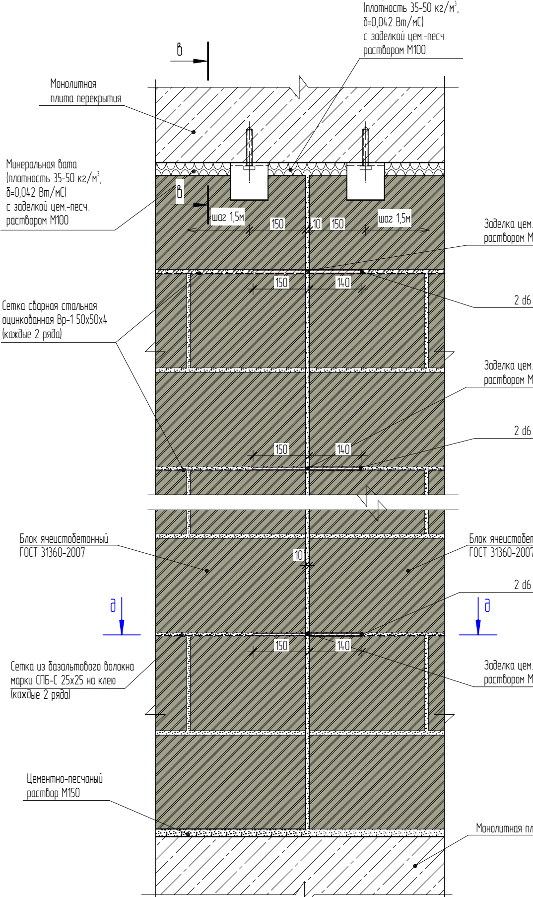
Вид В М110
