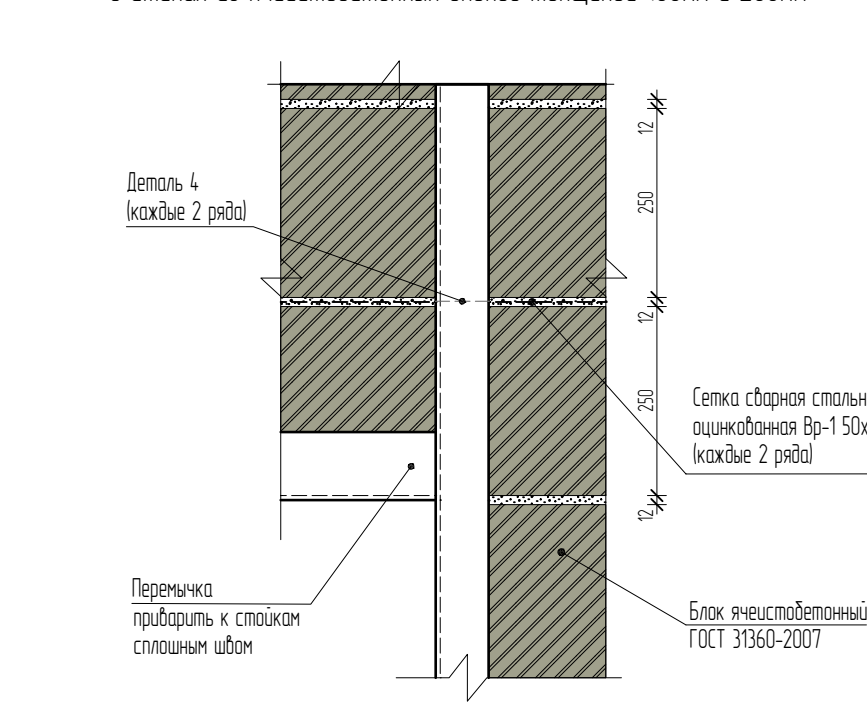
Вид Д2 М110
