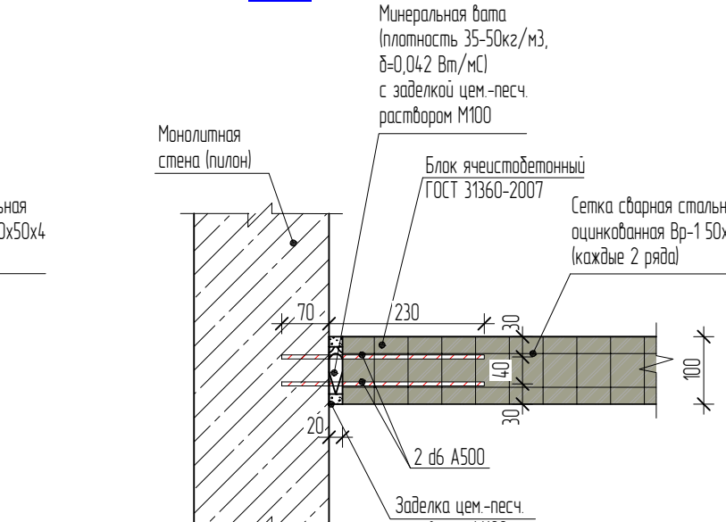
б1 - б1
