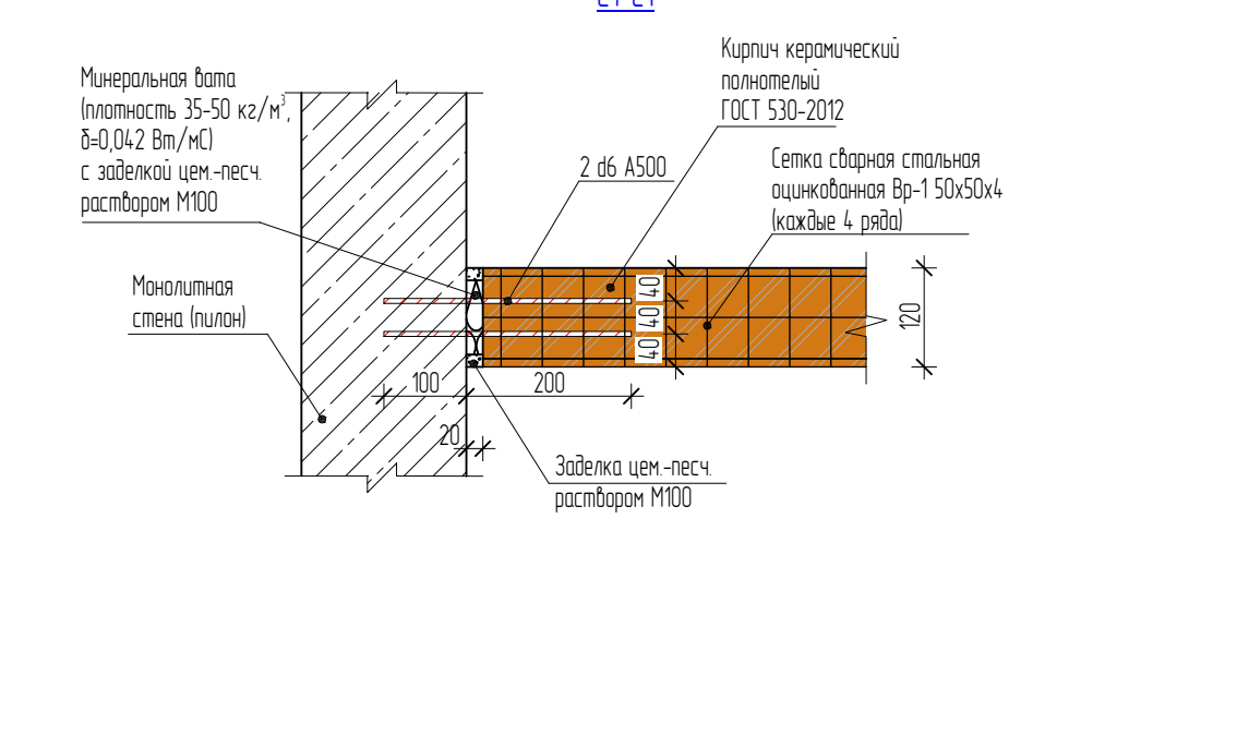
е1-е1
